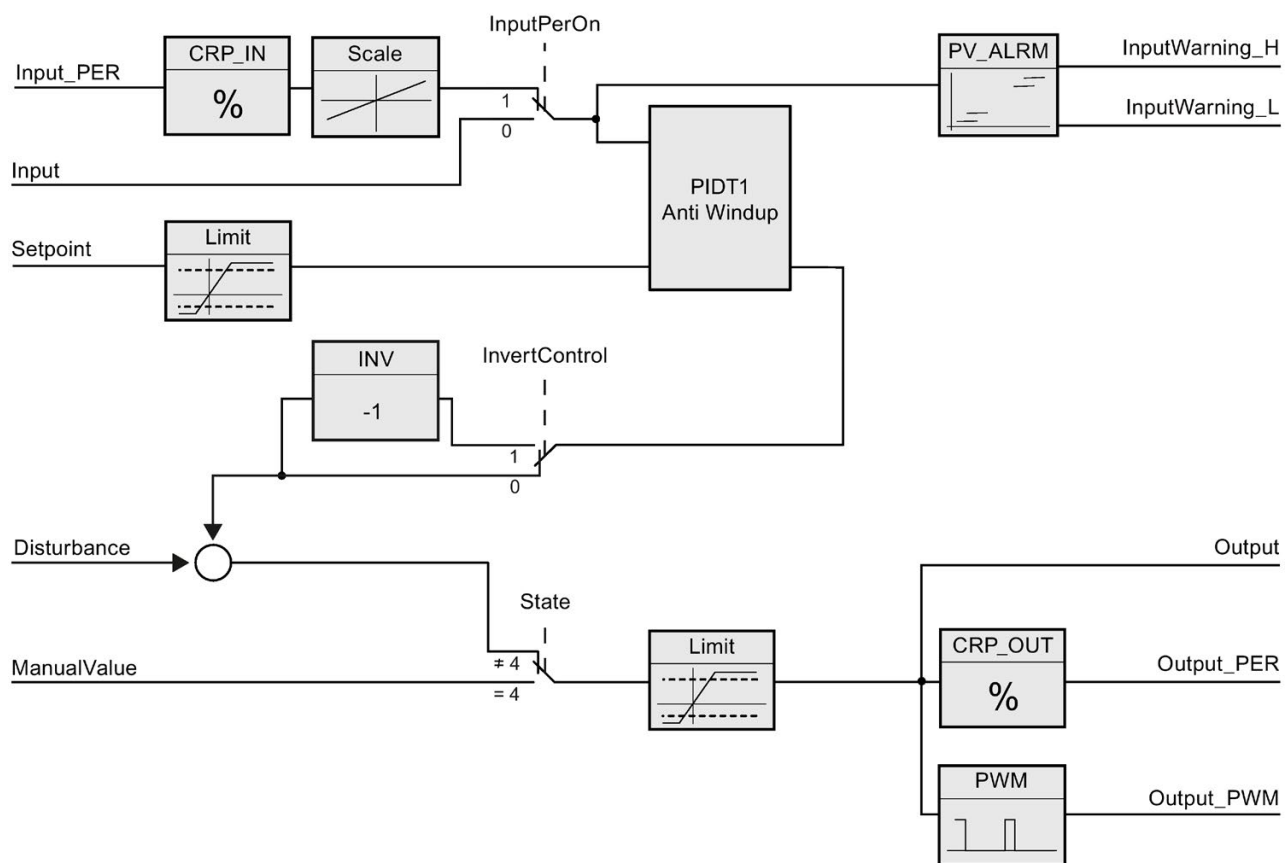
PID_Compact 方框图
