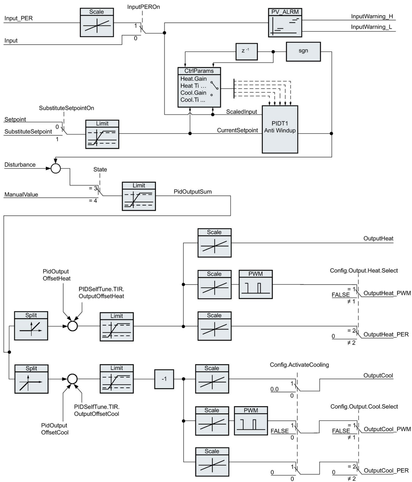
PID_Temp 方框图
