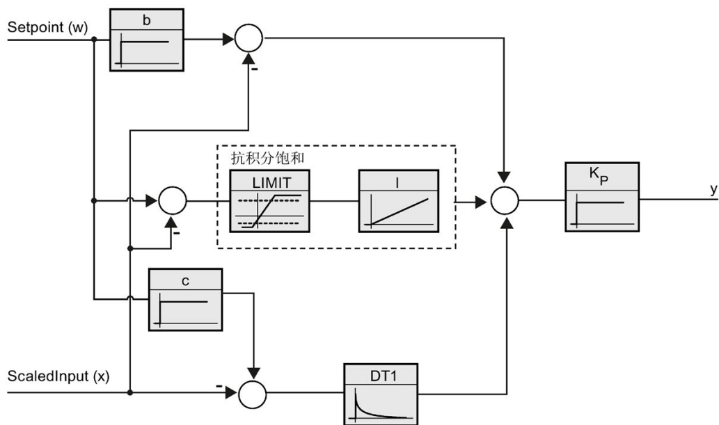
带抗积分饱和的 PIDT1 的方框图
