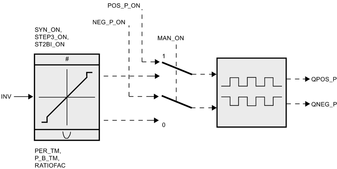
方框图
