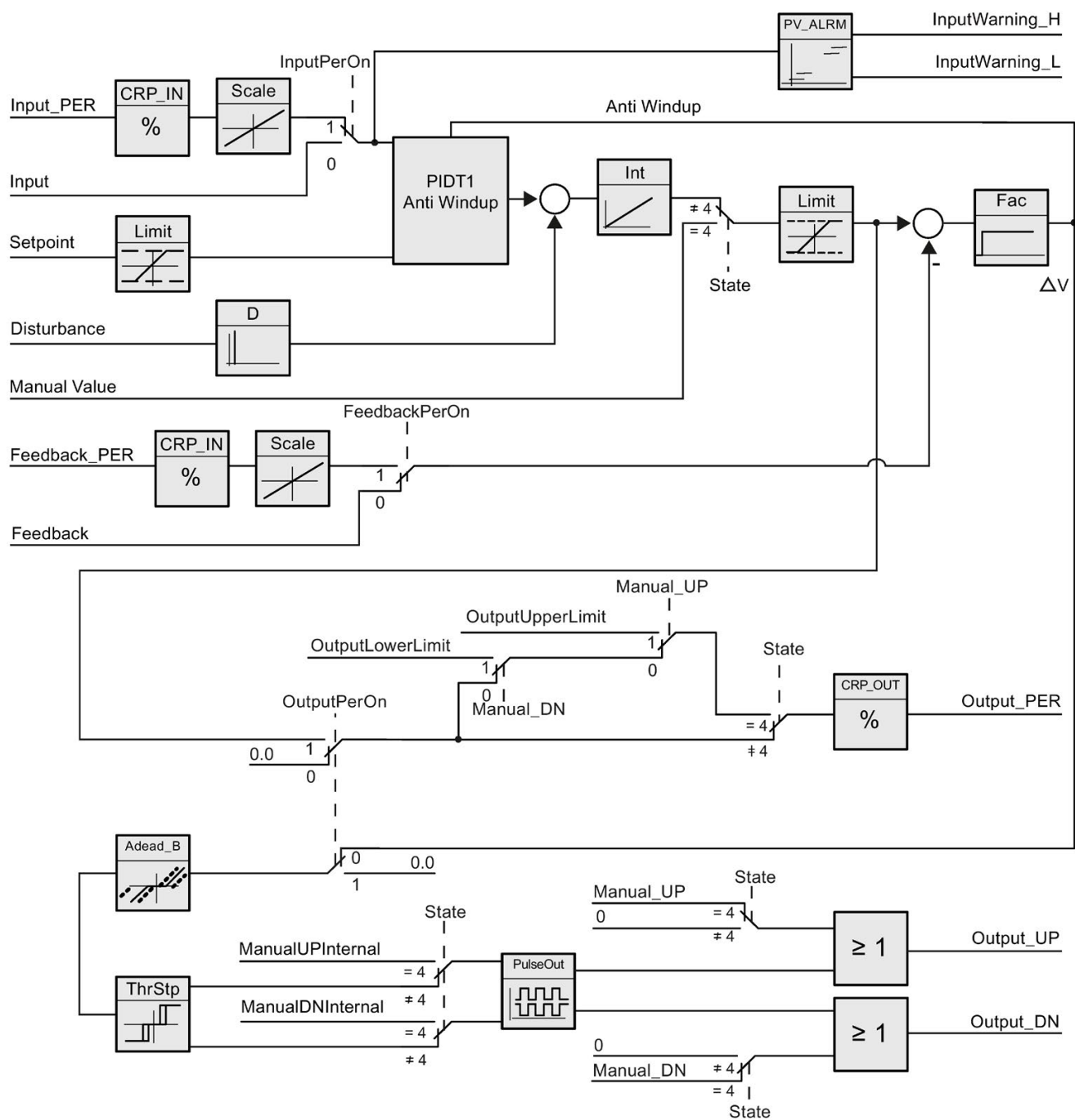
带位置反馈的方框图
