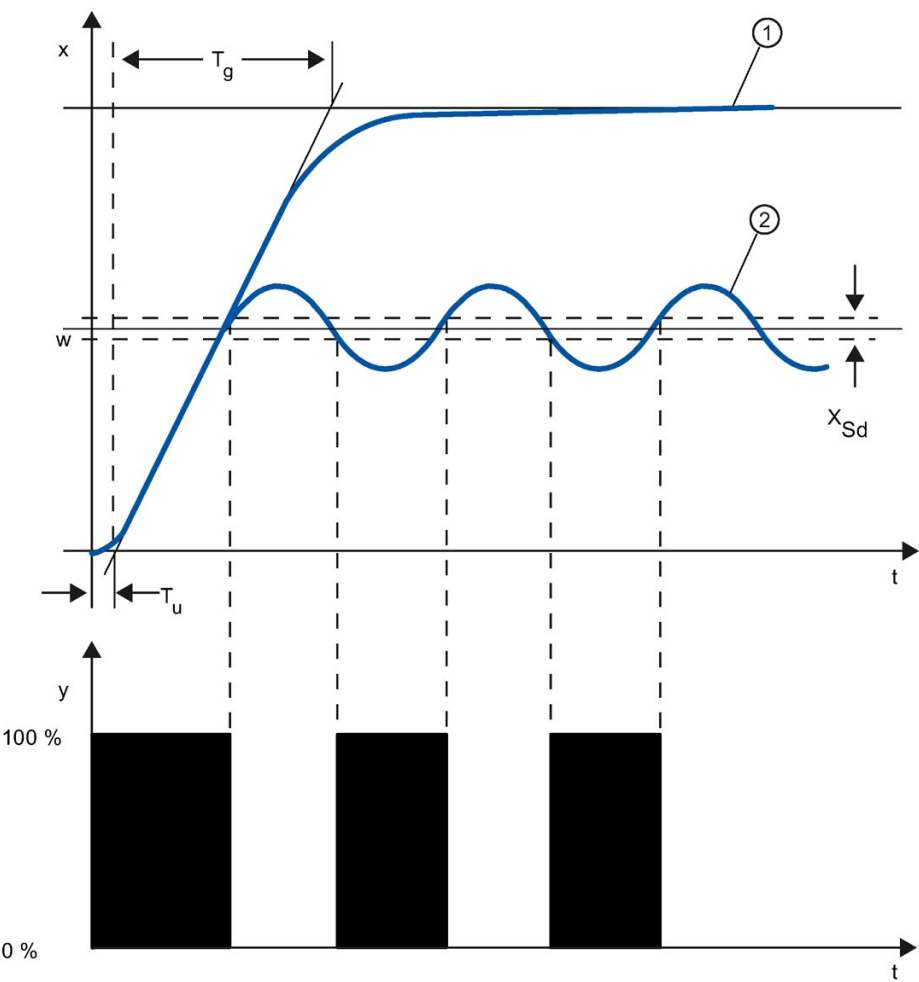
下图显示了两位控制器的控制函数
