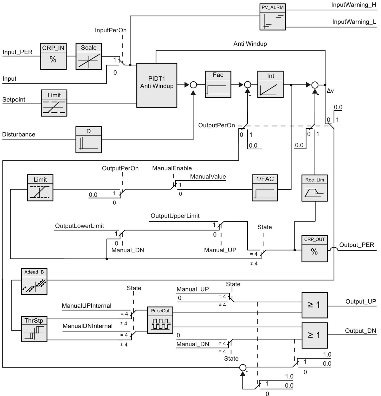
不带位置反馈的方框图
