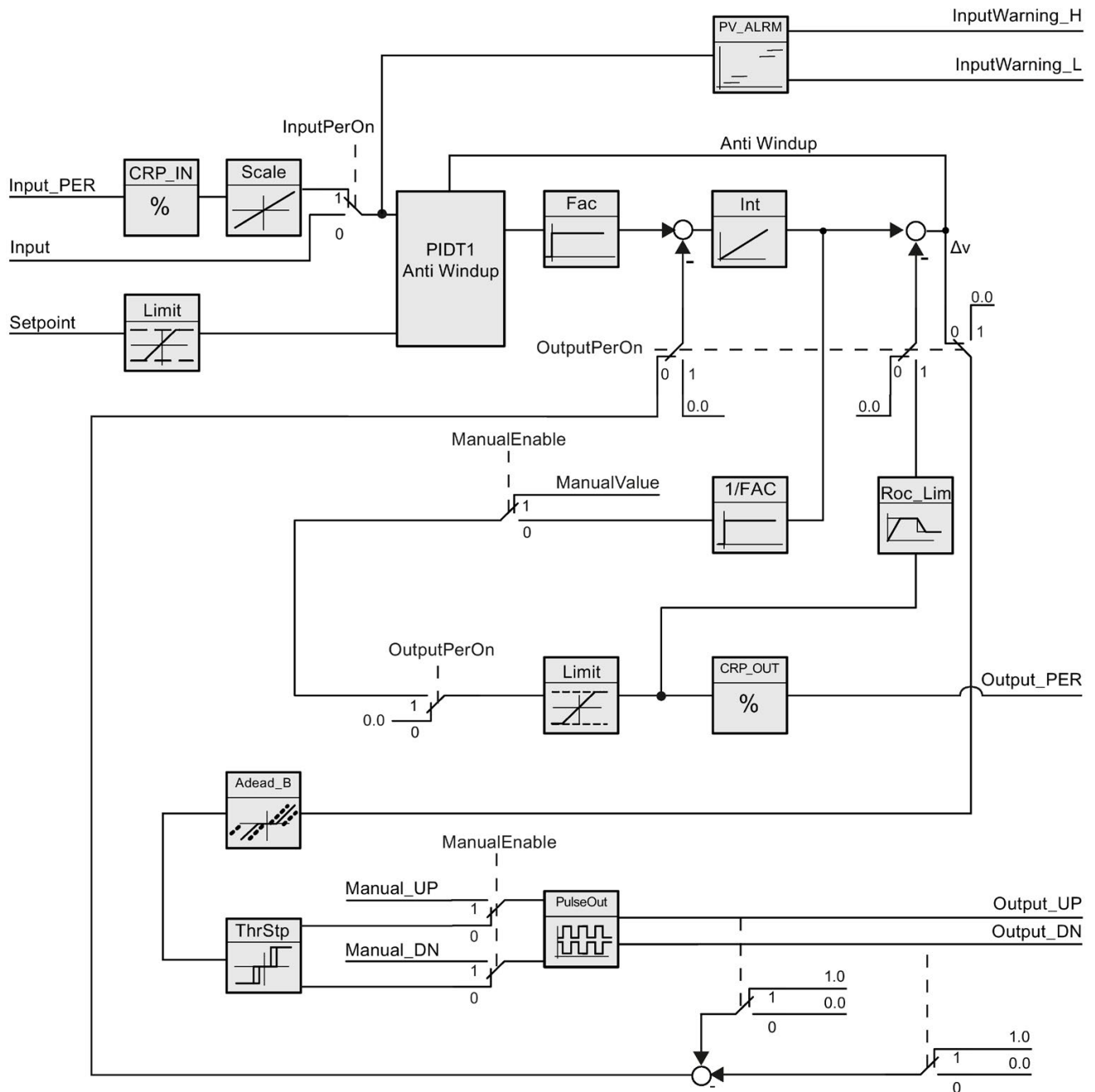
不帶位置反馈的方框图
