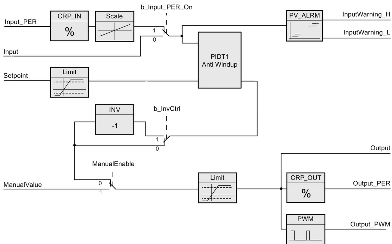
PID_Compact 方框图
