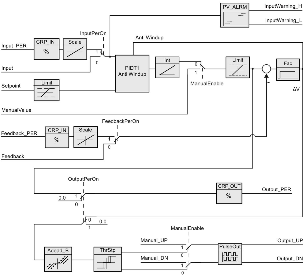
带位置反馈的方框图
