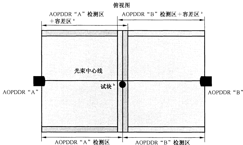
图 3g) 光干涉试验
