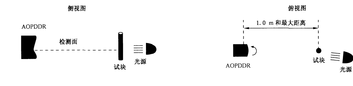
图 3a) 背景对检测能力的影响——例 1
