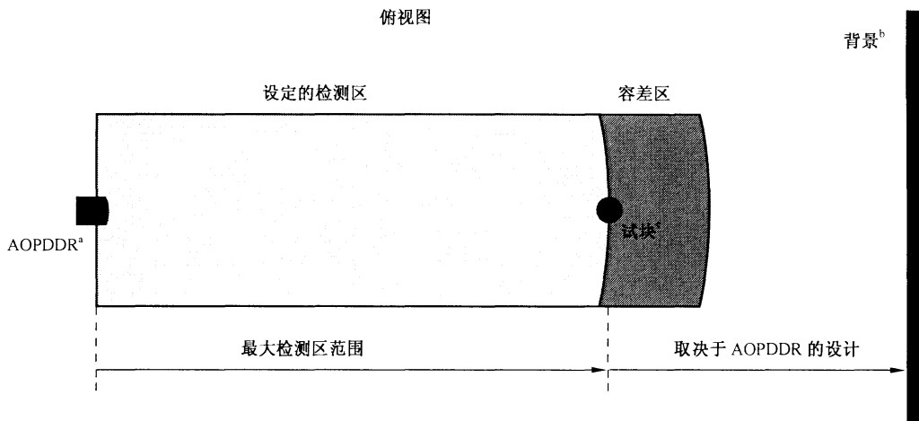
图 3h) 等同设计的两个 AOPDDRs 间的干涉
