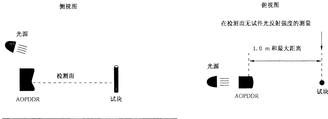
图 3d) 背景反射光对检测能力的影响
