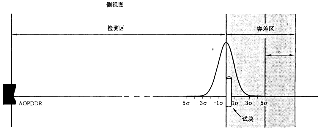
图 BB. 3 测距精度、检测区和公差带的关系——示例 1
