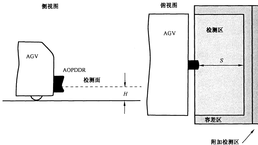
图 AA.2 AOPDDR 在 AGV 上使用的示例
