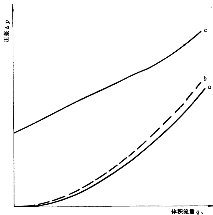
图 12 液控单向阀稳态压差-流量特性曲线
