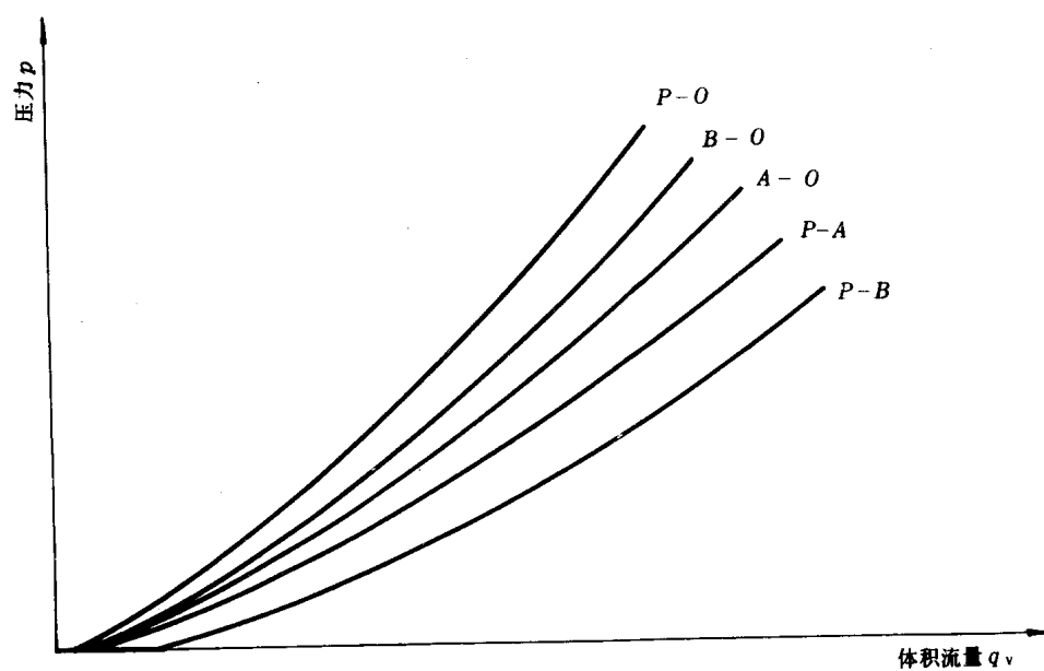
图 2 稳态压差—流量特性曲线
