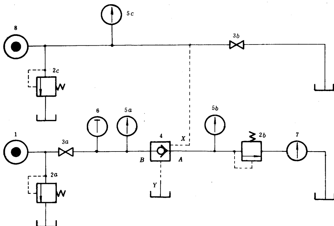
图 11 液控单向阀试验回路
