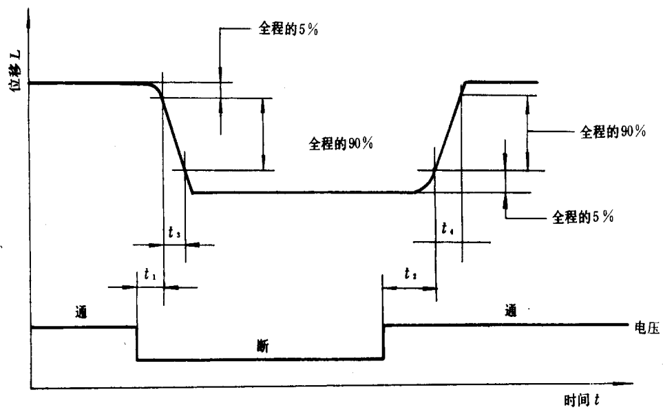
a 阀芯位移-时间关系曲线
