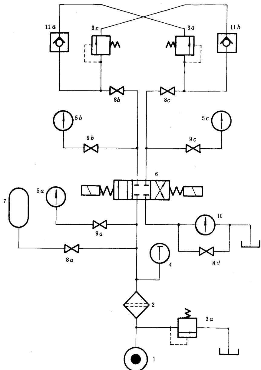
图 1 电磁换向阀试验回路
