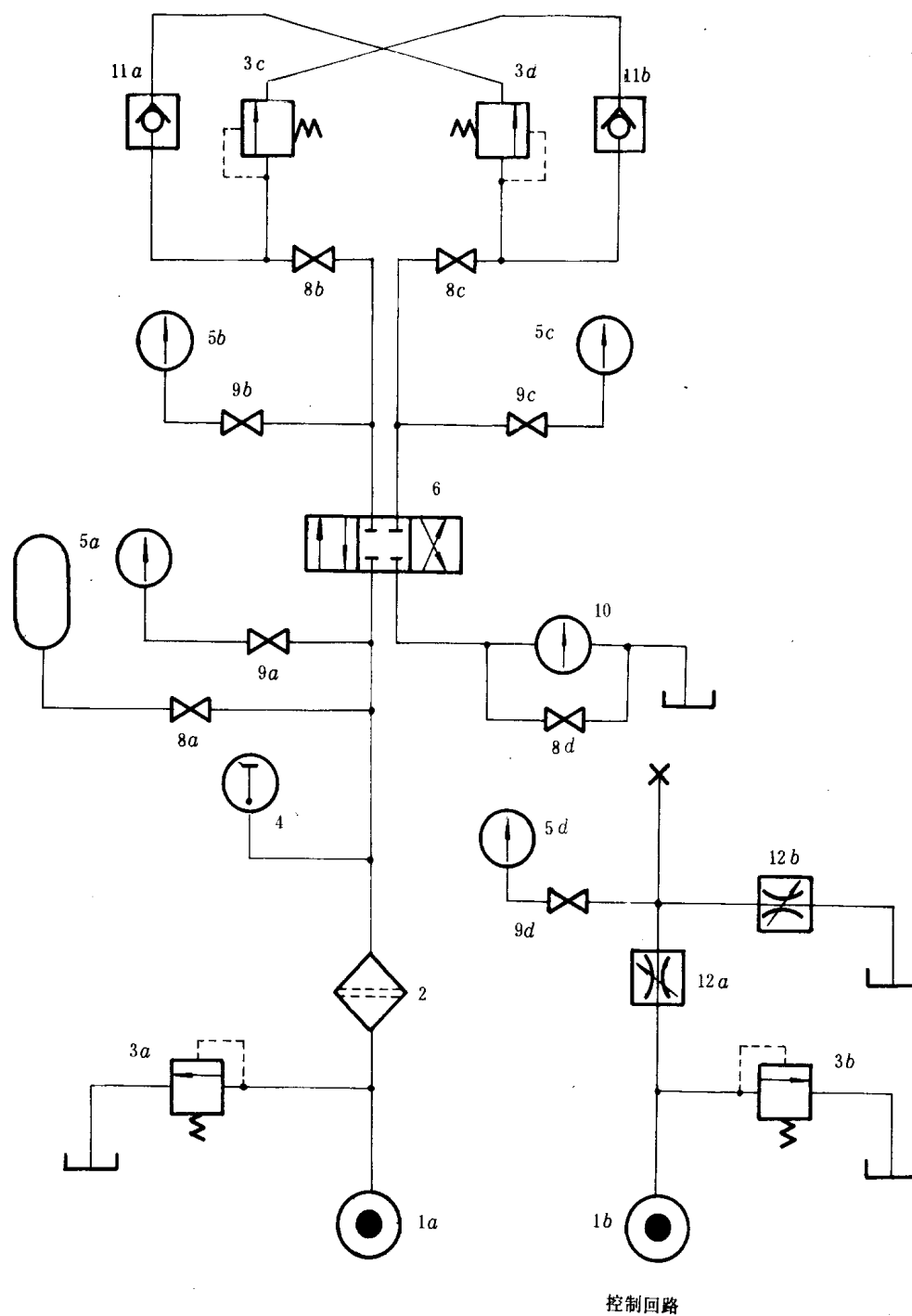
图 8 电液换向阀、液动换向阀、手动换向阀试验回路
