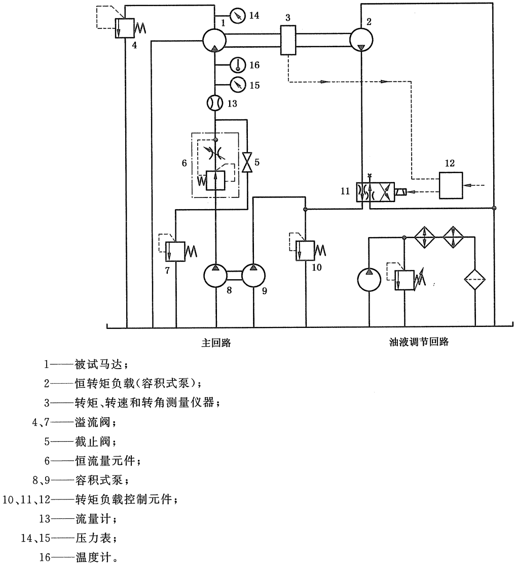
图 1 液压试验回路
