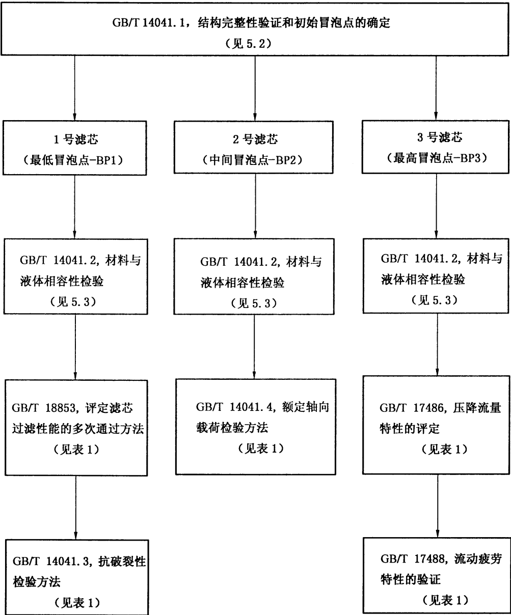
图 1 试验程序
