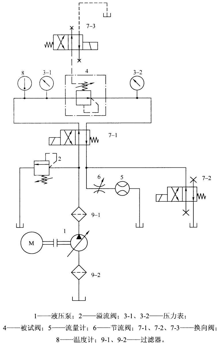
图 B.1 出厂试验回路原理图
