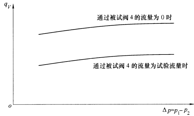
图 B.5 进口、出口压差-外泄漏量曲线
