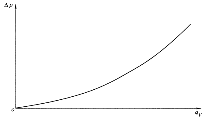
图 B.6 流量-反向压力损失曲线
