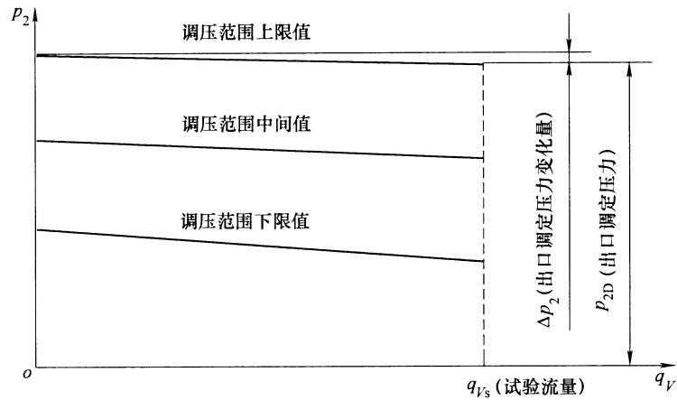
图 B.4 流量变化-出口调定压力变化特性曲线
