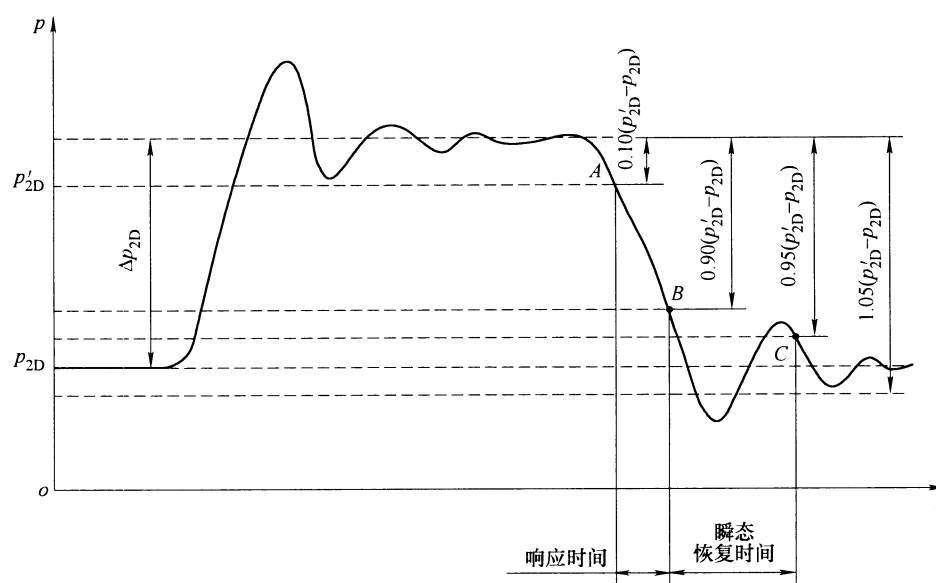
图 B.10 流量阶跃变化时被试阀 4 的出口调定压力响应特性曲线
