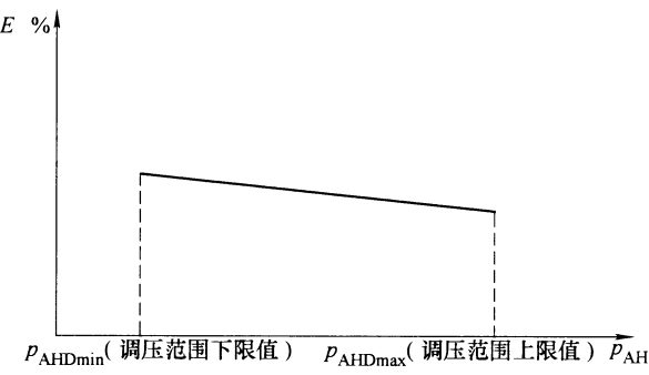
图 B.5 工作油口（A 口）调定压力-重复精度误差特性曲线
