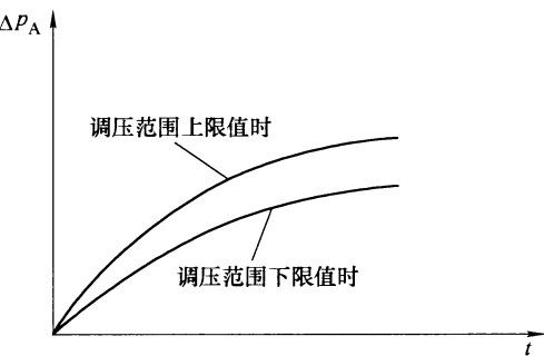
图 B.8 保压时间-工作油口（A 口）压降特性曲线
