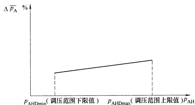
图 B.2 工作油口（A 口）调定压力-工作油口（A 口）压力变化率特性曲线
