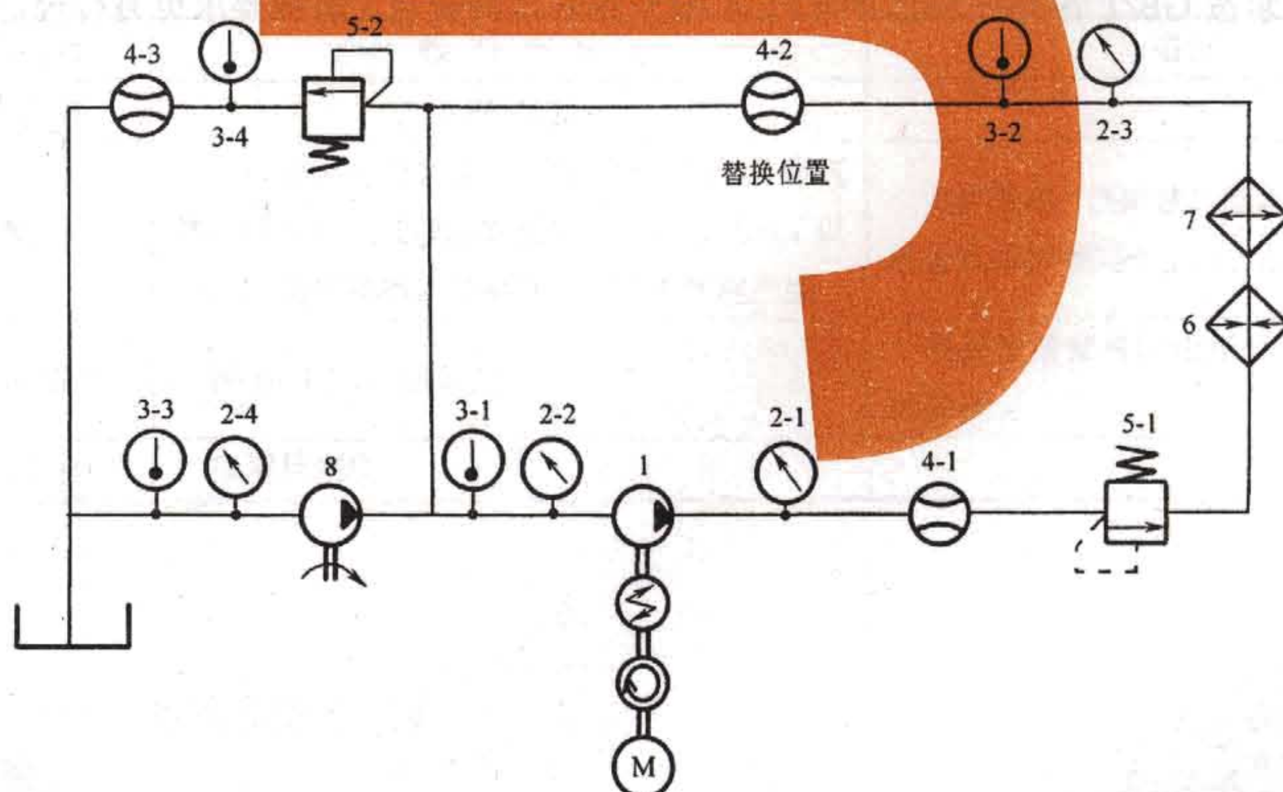
图 A.1 开式试验回路原理图
