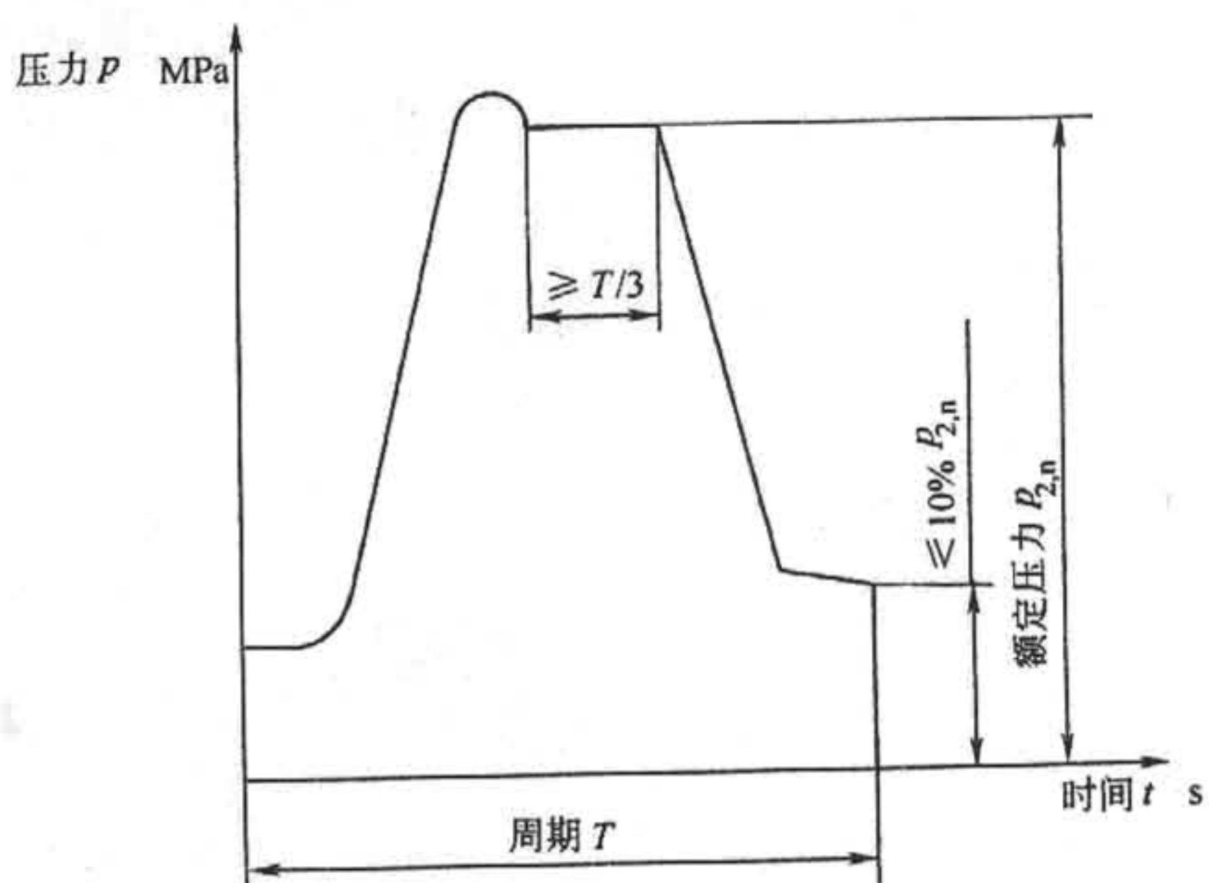
图 A.6 冲击波形
