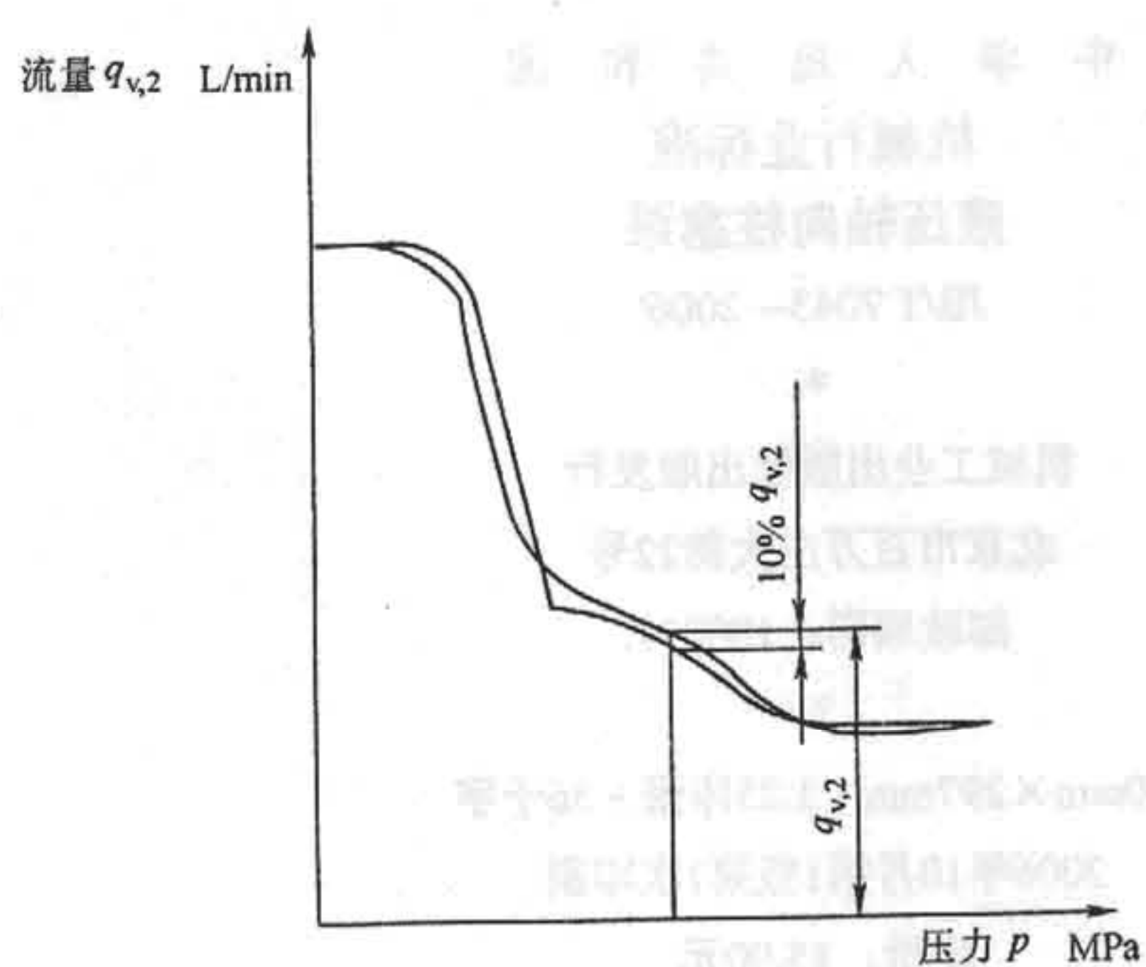
图 A.5 恒功率特性曲线
