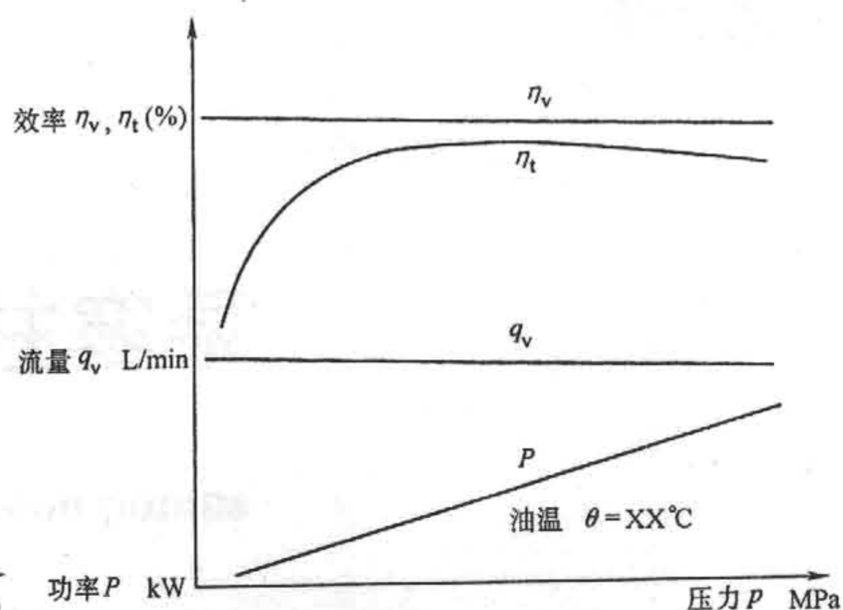
图 A.4 功率、流量、效率随压力变化曲线
